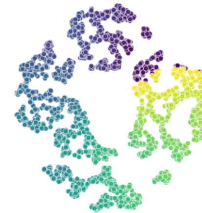
t-SNE
