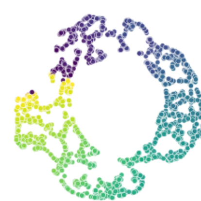
UMAP
