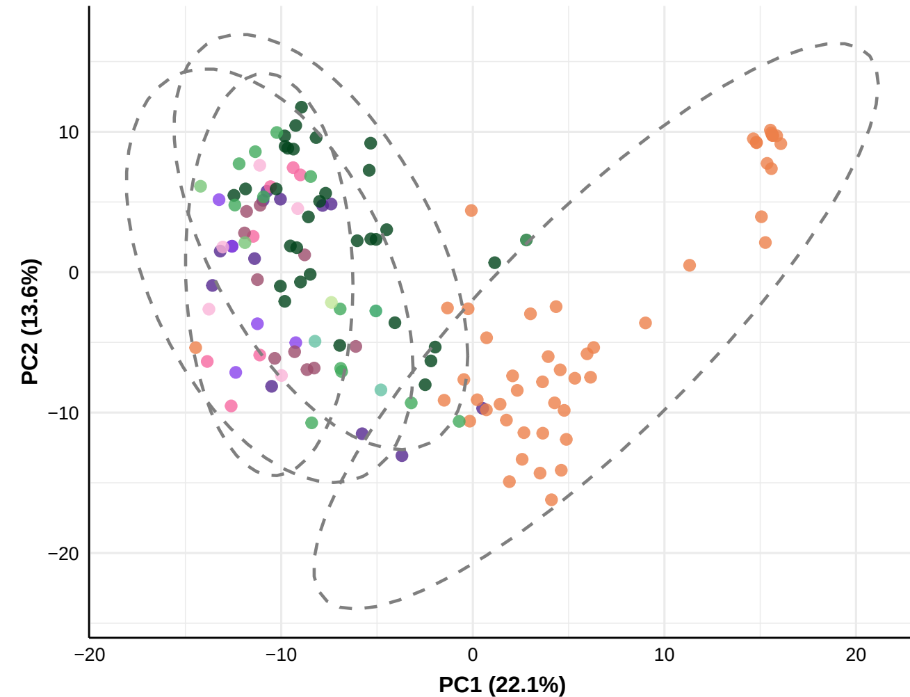
A) Control: Lipid PCA
