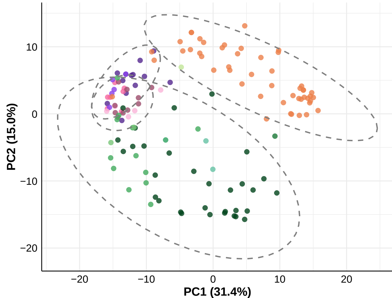
B) LowInput: Lipid PCA
