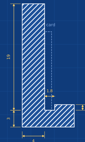
SECTION D-D (3:1)
