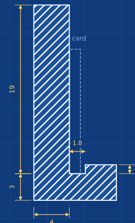
SECTION D-D (3:1)
