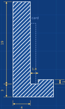
SECTION D-D (3:1)
