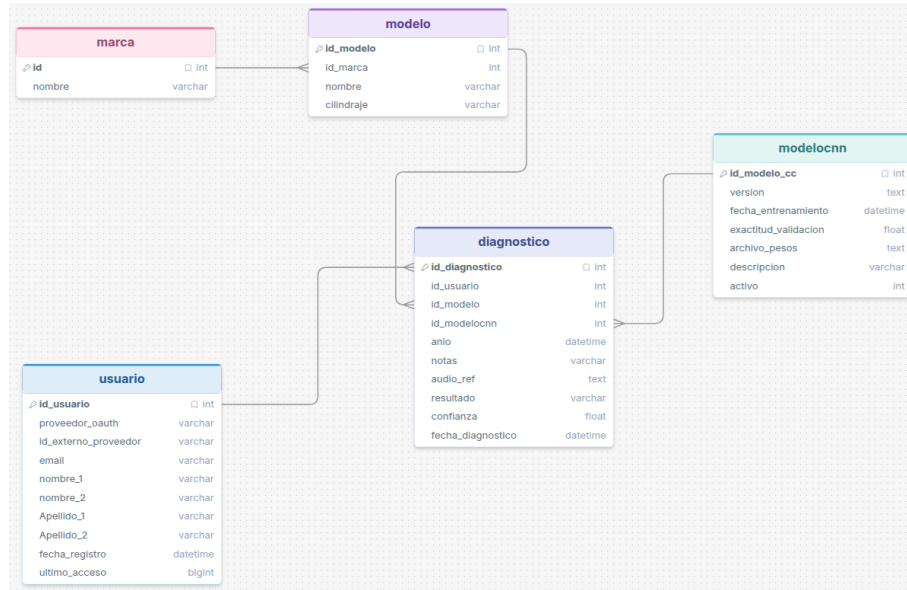
Figura 4: Diagrama entidad-relación (3NF)
