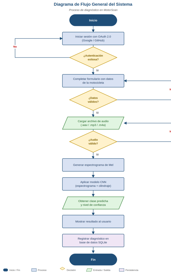
Figura 8: Diagrama de flujo general
