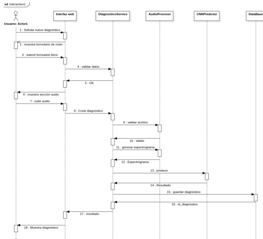
Figura 6: Diagrama de secuencia
