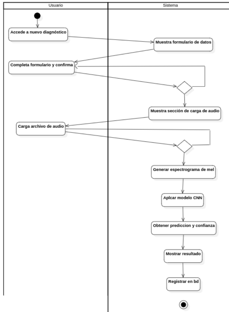
Figura 7: Diagrama de actividades
