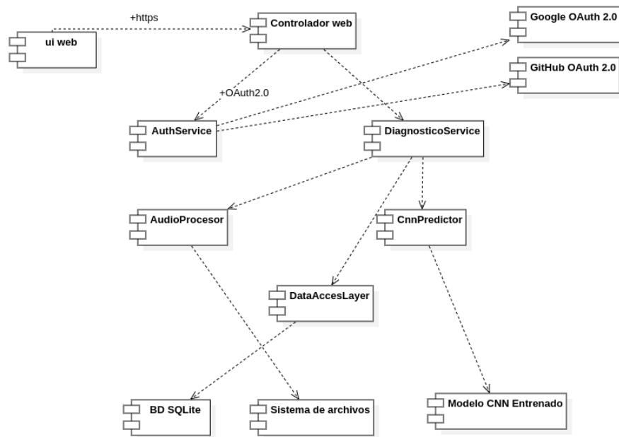
Figura 2: Diagrama de componentes
