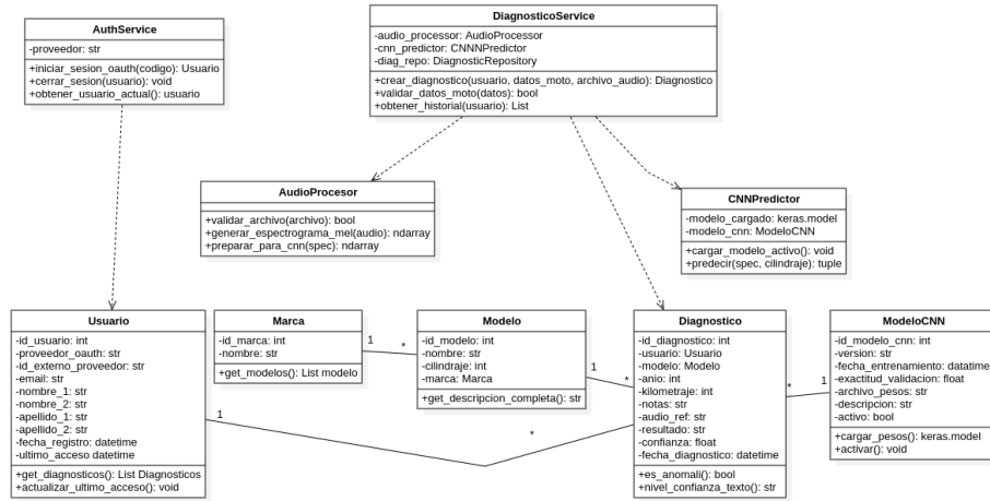
Figura 5: Diagrama de clases
