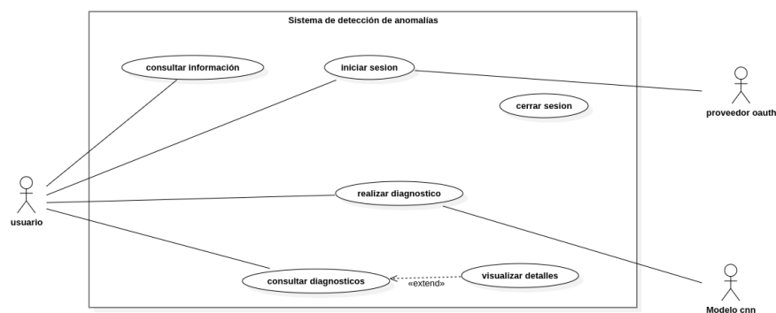
Figura 1: Diagrama de casos de uso
