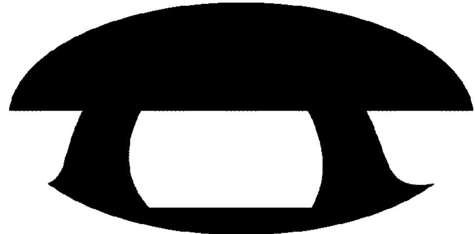
Survey mask
