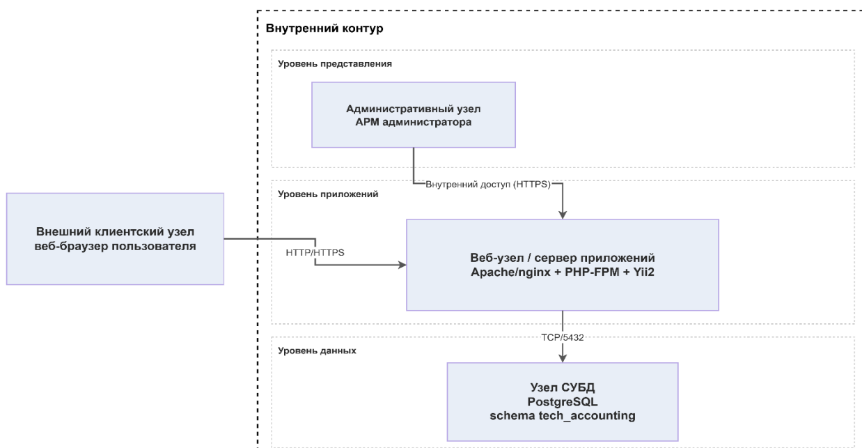
Рисунок 2.3 — UML-диаграмма развёртывания прототипа
