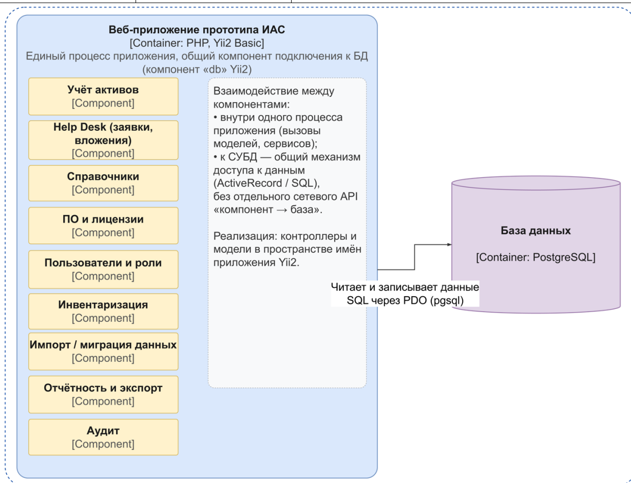
Рисунок 2.2 — Логические компоненты и контейнеры доступа к данным
