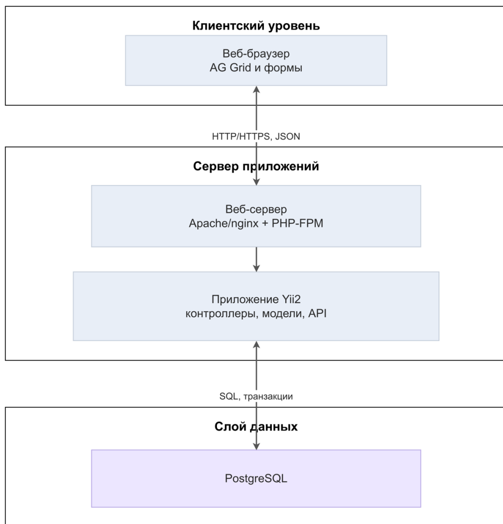
Рисунок 2.1 — Многослойная клиент-серверная архитектура прототипа ИАС
