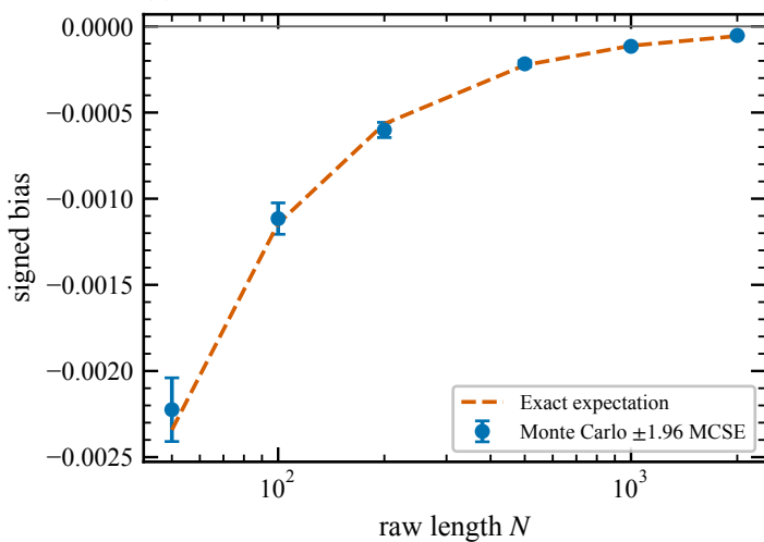
(d) U : simulation and exact value, m = 4
