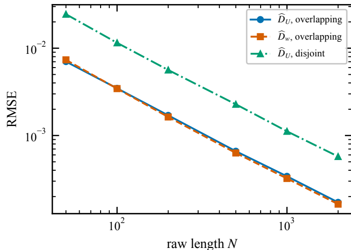
(d) Common local scale, white noise m = 5
