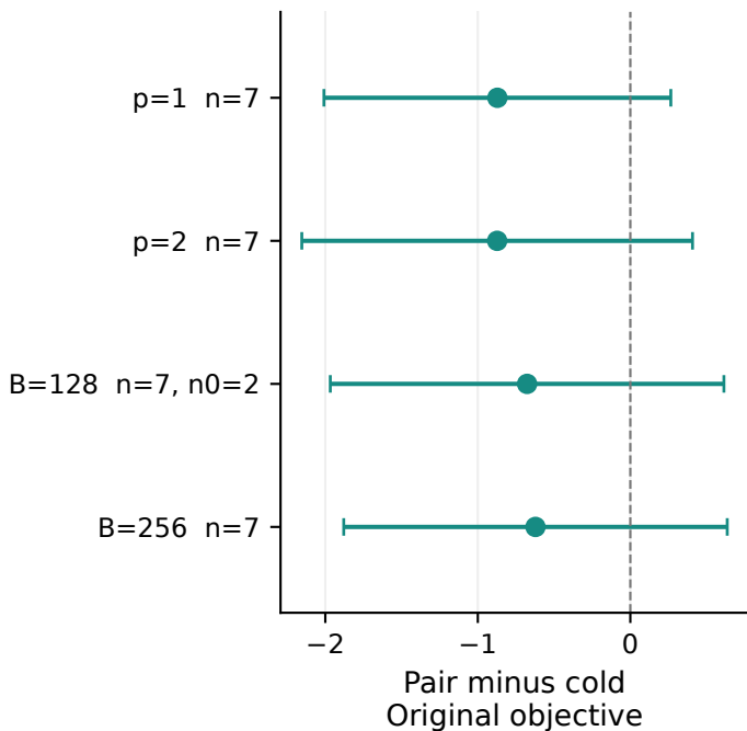
Max-3SAT
