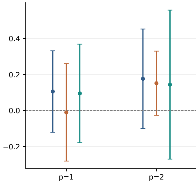
Cubic spin glass (n=10)
