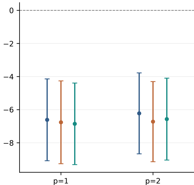
Max-3SAT (n=10)
