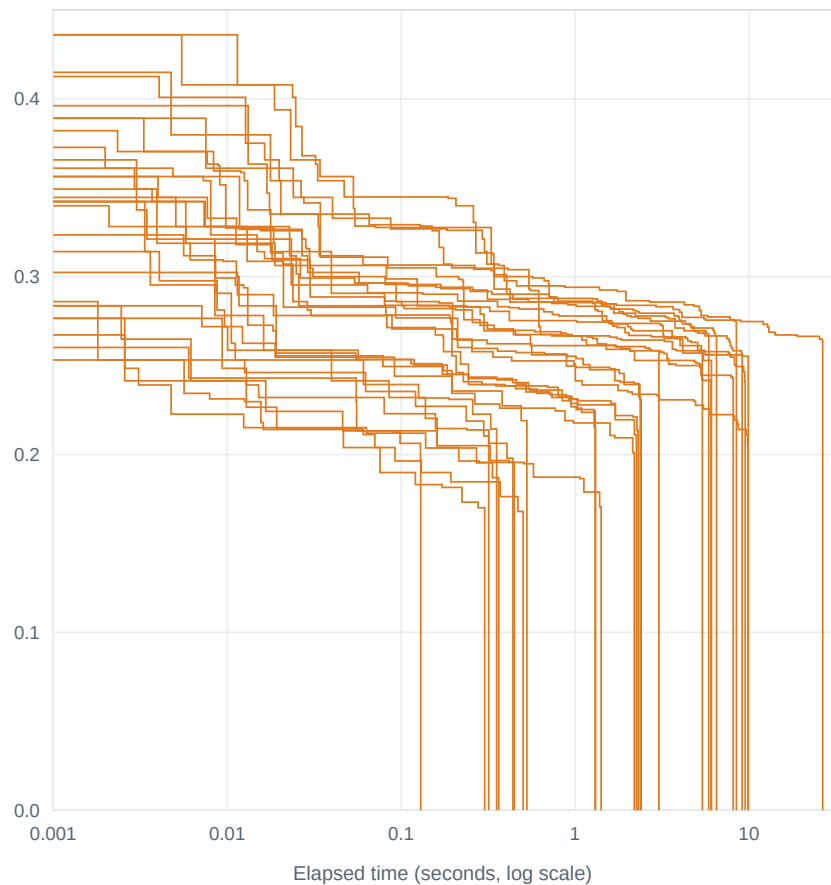
Max-3SAT (N=30)
