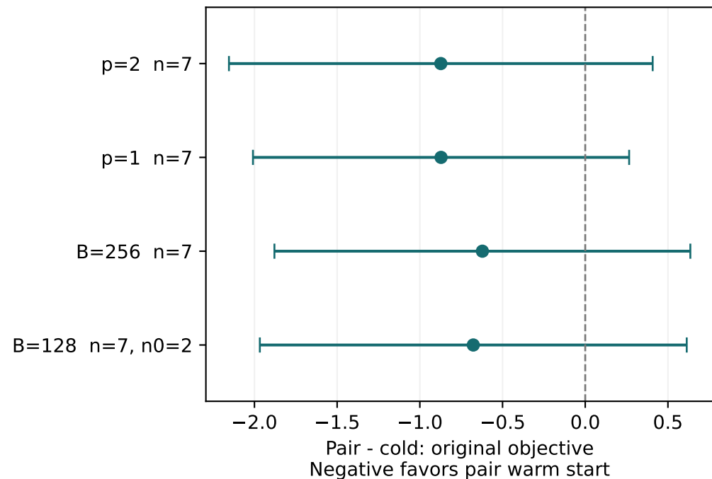
Max-3SAT
