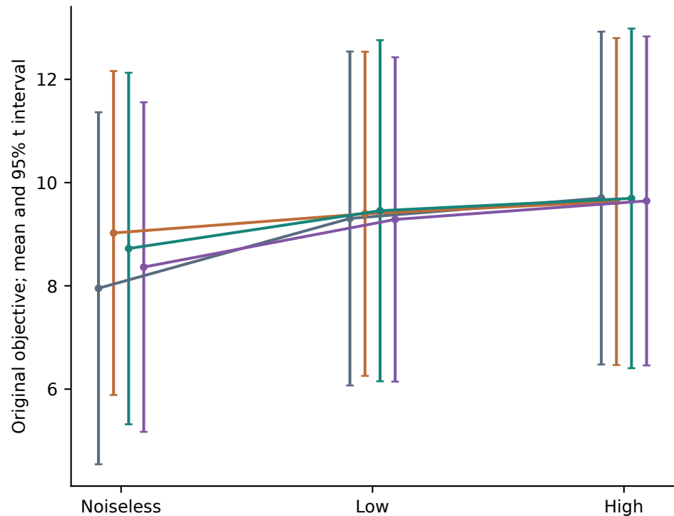
Max-3SAT | n=9
