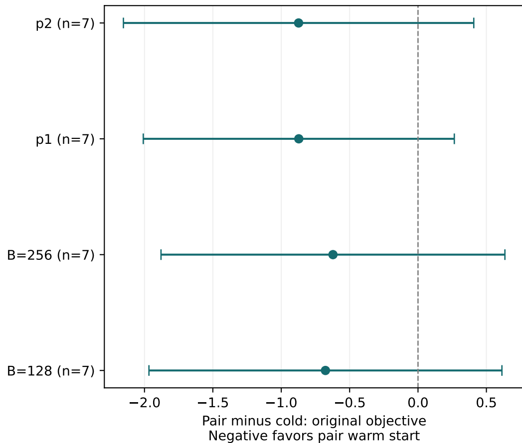
Max-3SAT
