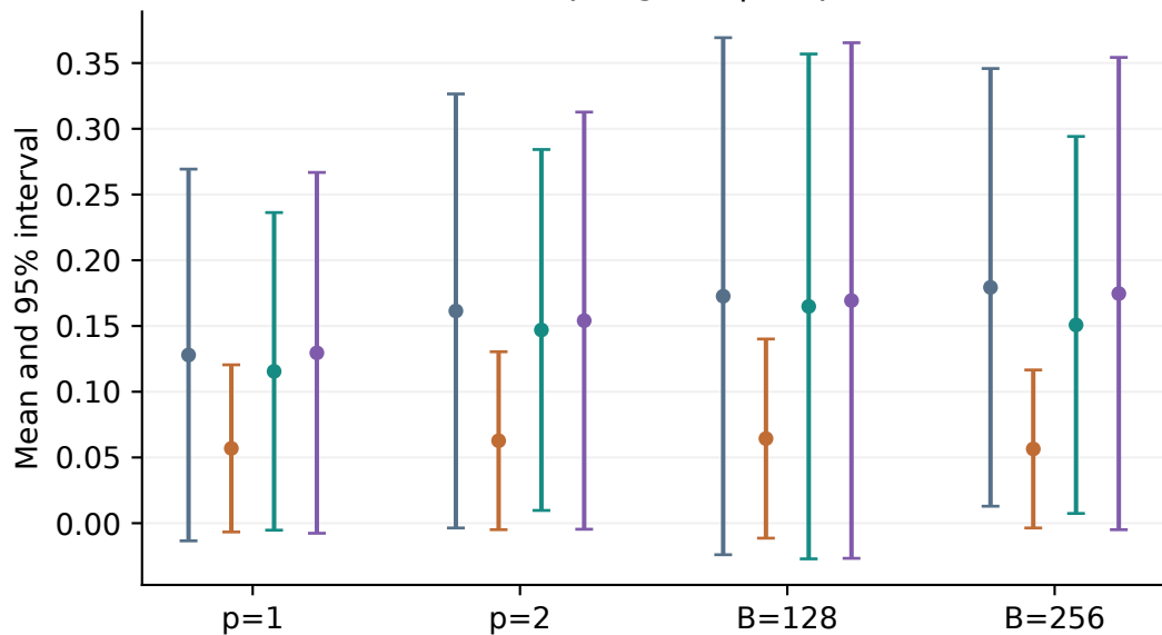
Max-3SAT | P(opt)
