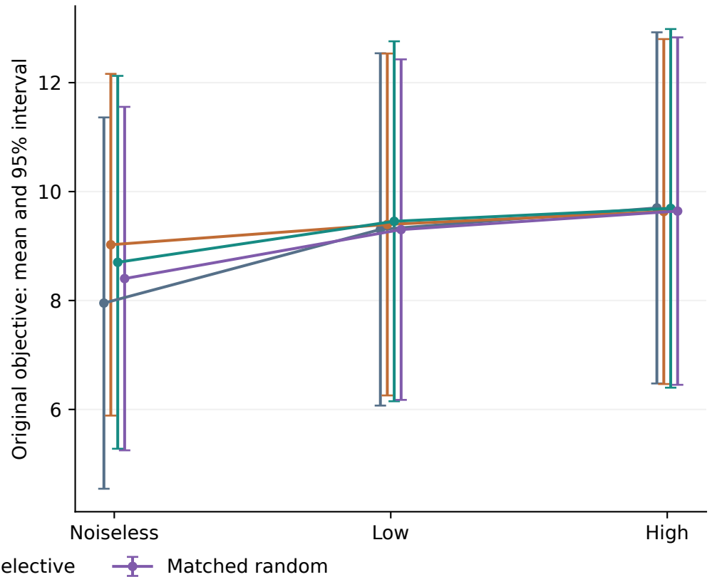
Max-3SAT | n=9
