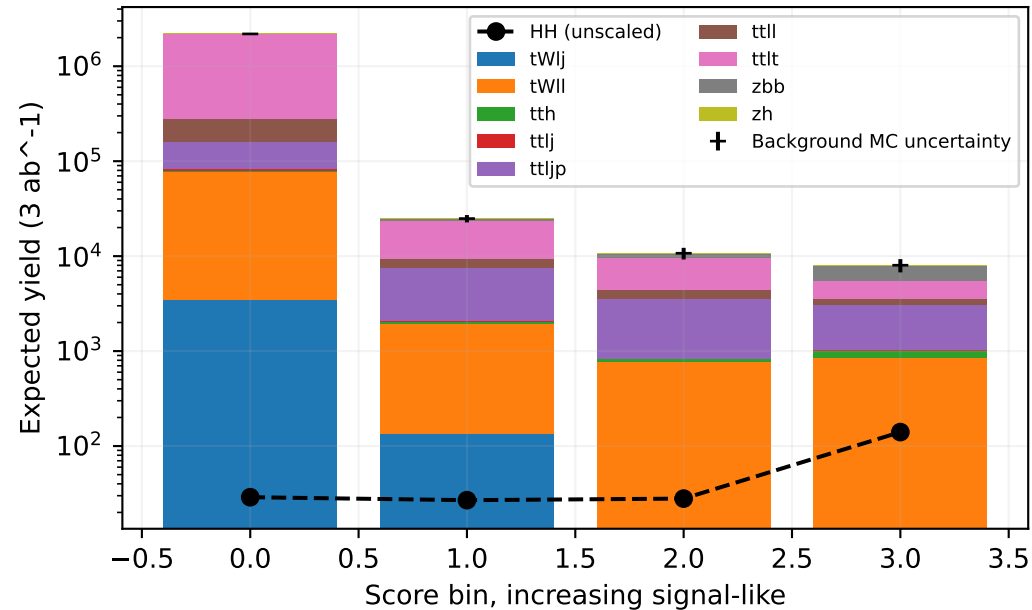
SLT Hi: m_{HH} > 350 \text{ GeV}
