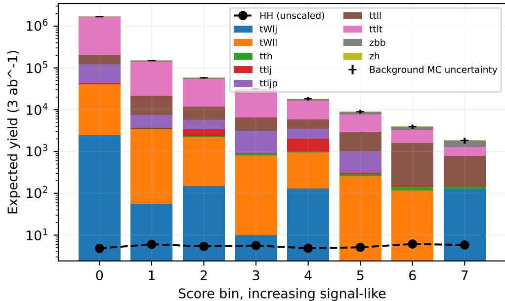
SLT Lo: m_{HH} \leq 350 \text{ GeV}
