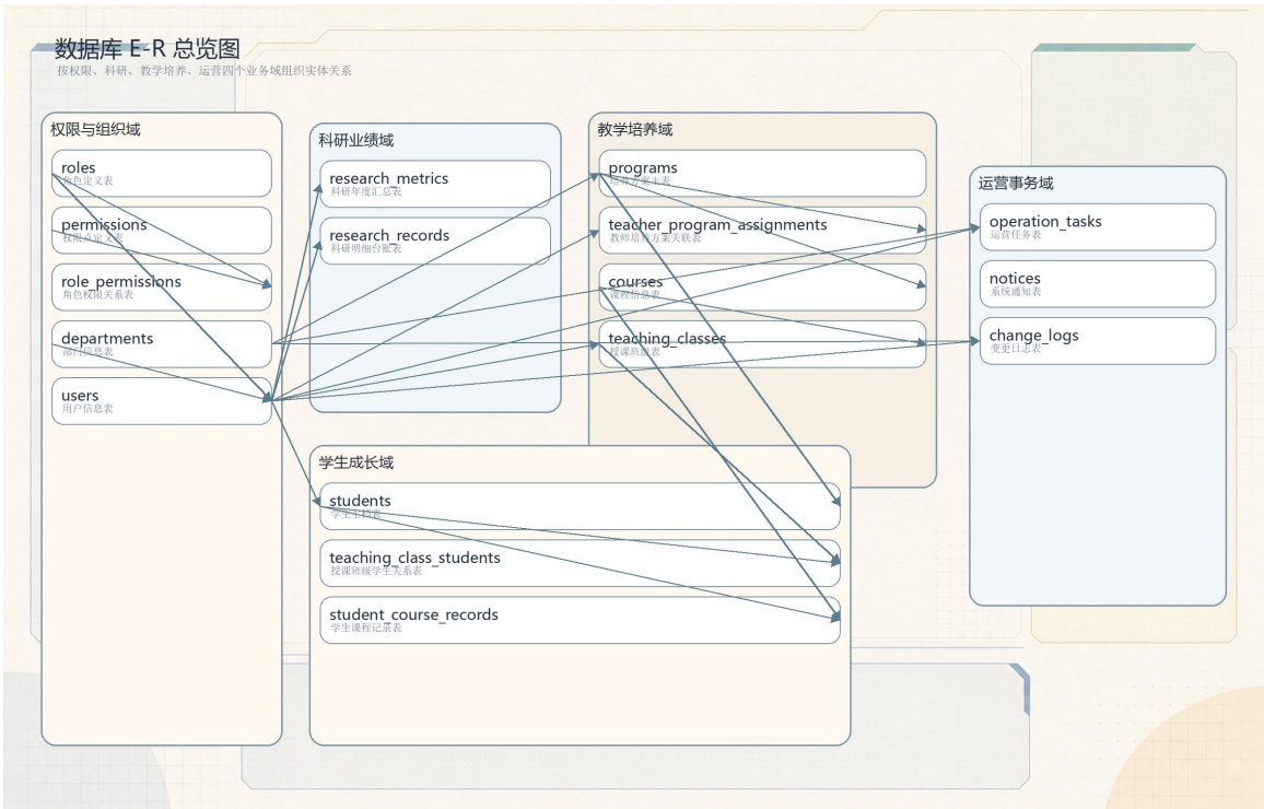
图 6-1 数据库 E-R 总览图
