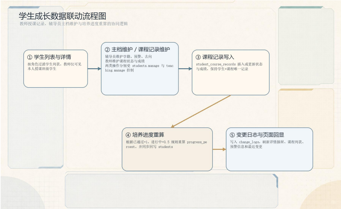
图 4-2 学生成长数据联动流程图
