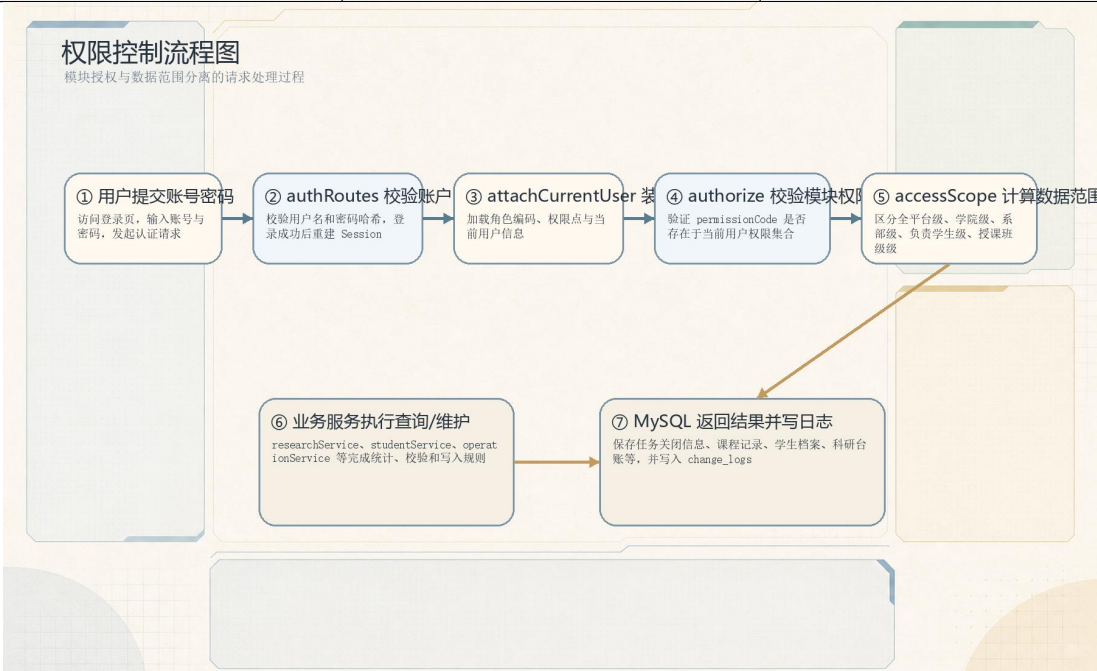
图 4-1 权限控制流程图
