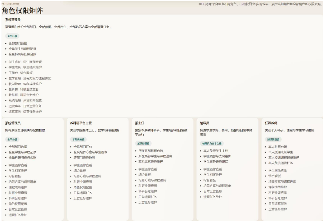
图 4-5 权限矩阵页面
