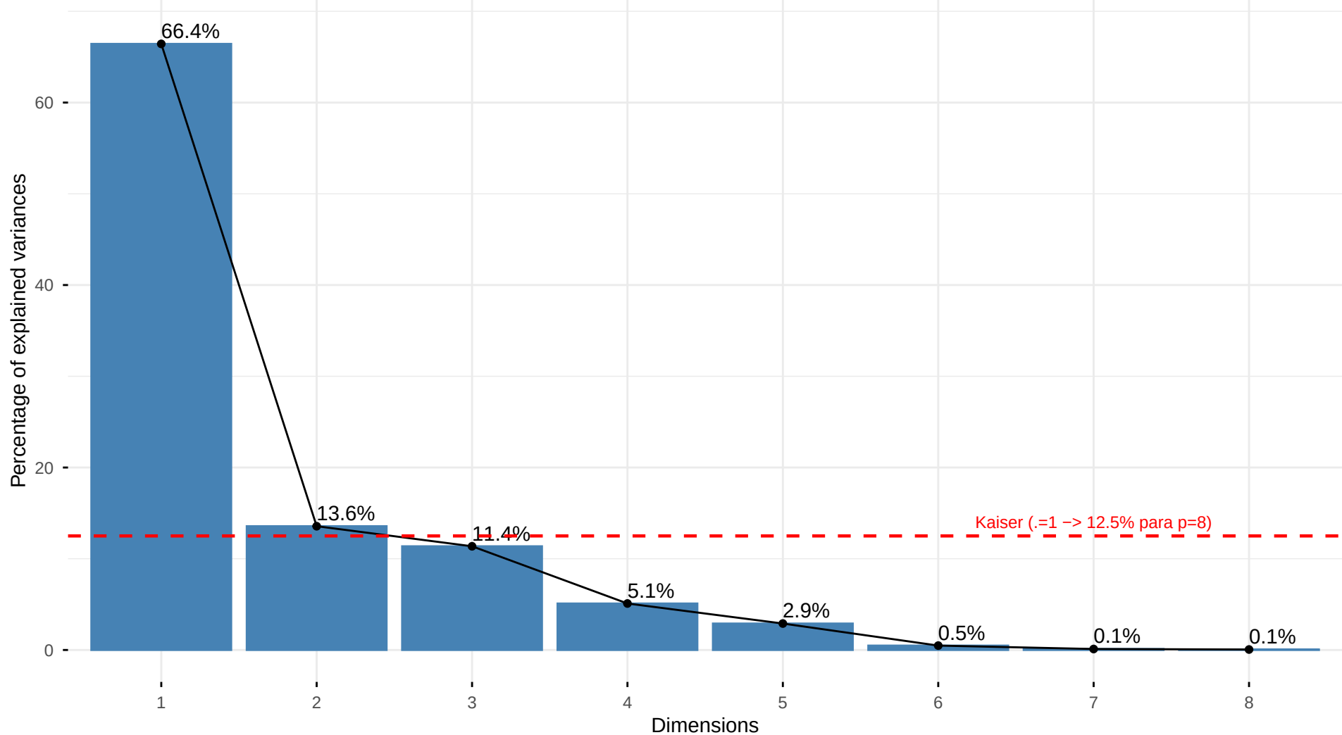
Scree Plot – Escolha de Componentes (Regra do Cotovelo)
