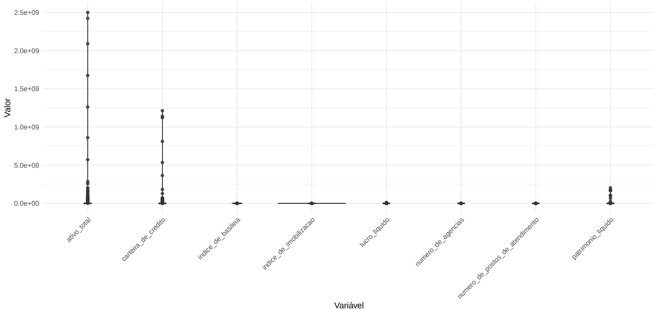
Violin Plots – Densidade das Distribuições
