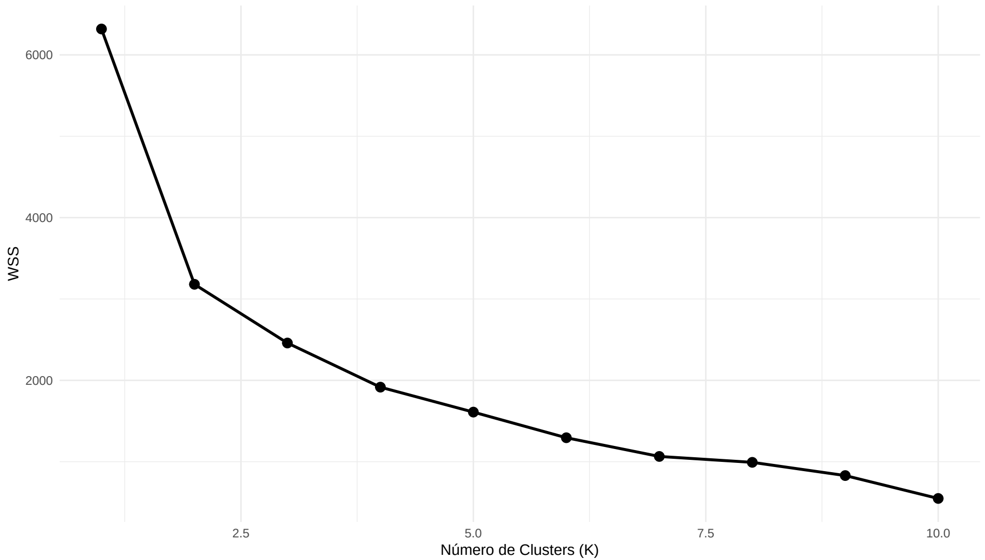
Método do Cotovelo – Sem Big 5
