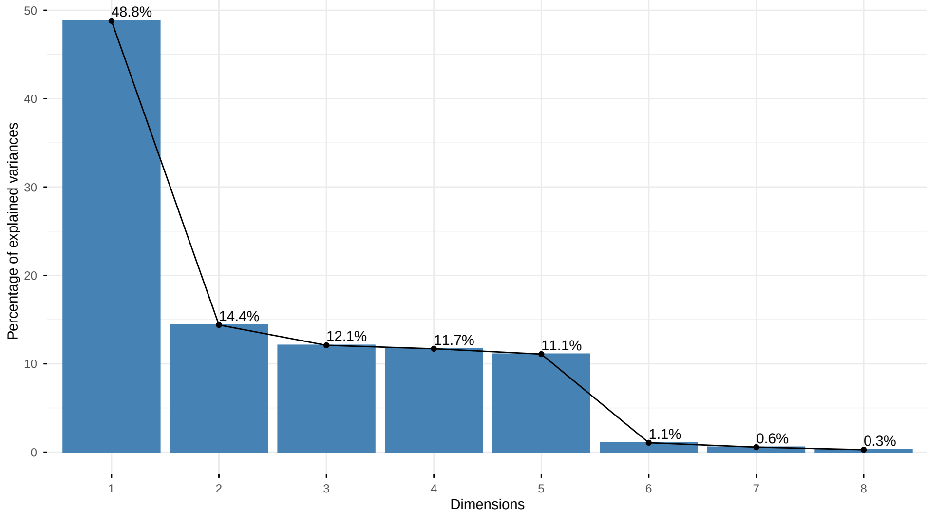
Scree Plot – PCA sem Big 5
