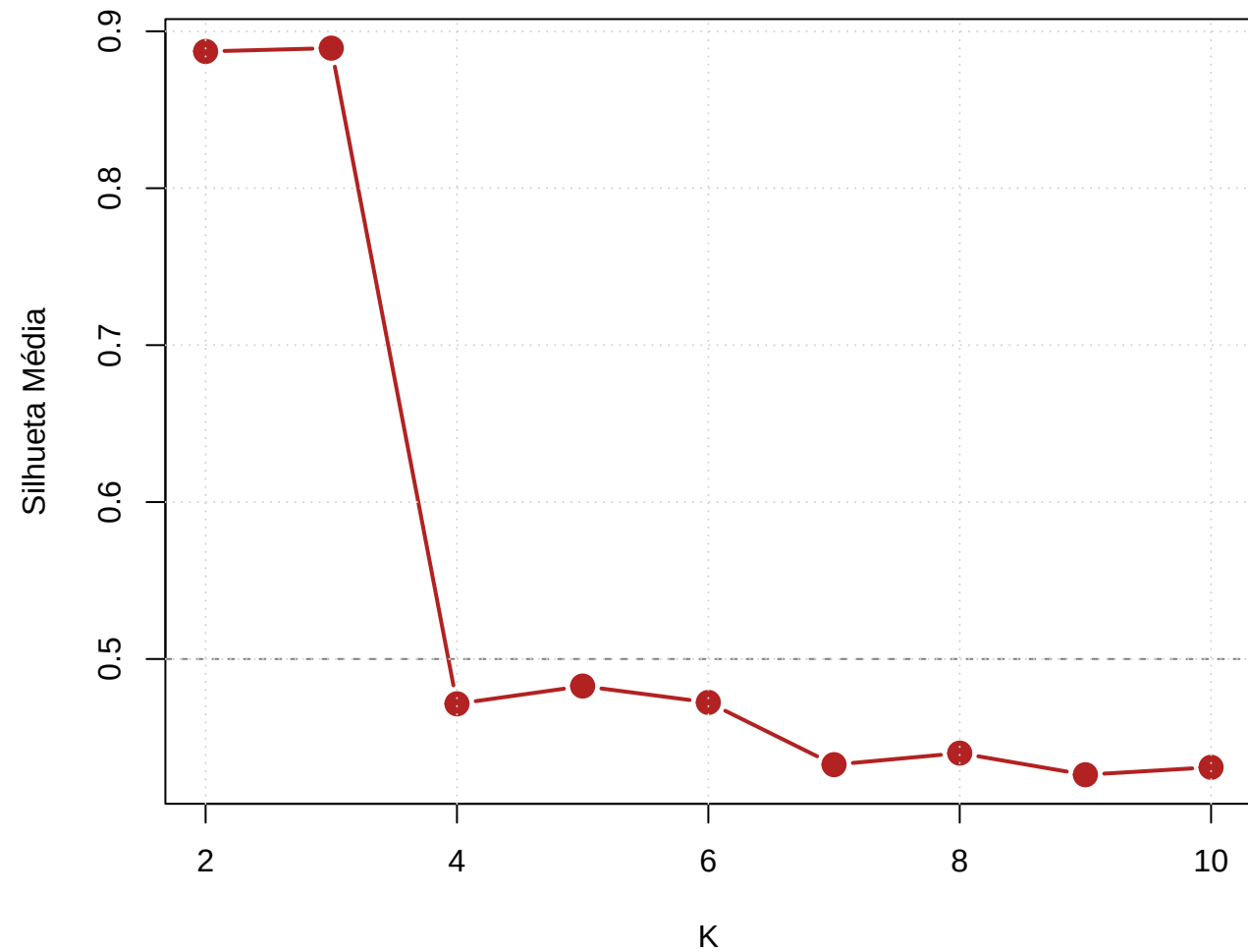
Coeficiente de Silhueta (sem Big 7)
