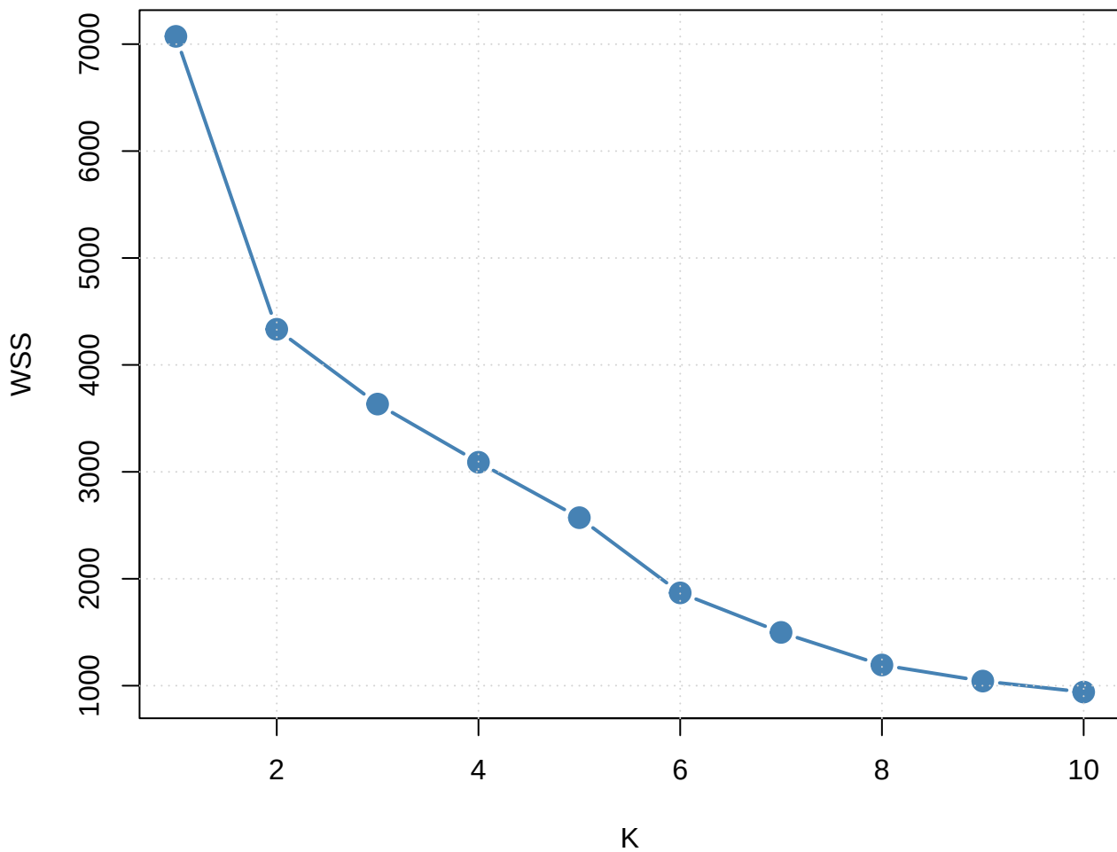
Método do Cotovelo (sem Big 7)
