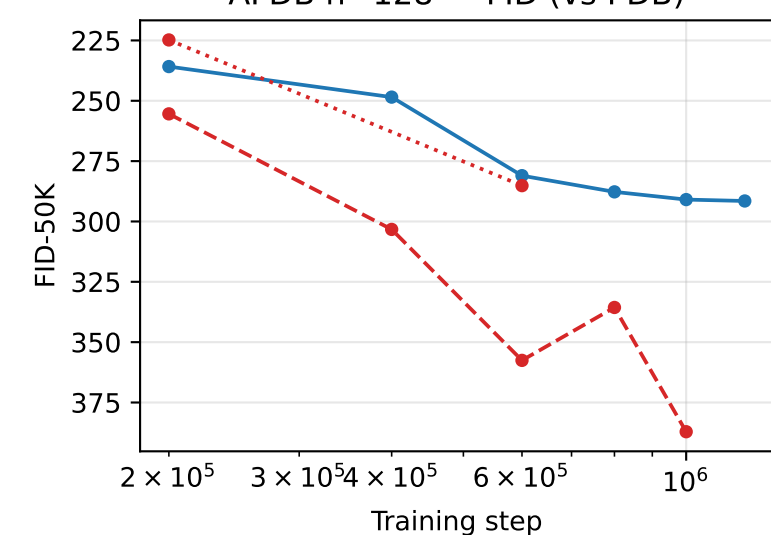
AFDB n=128 — FID (vs PDB)
