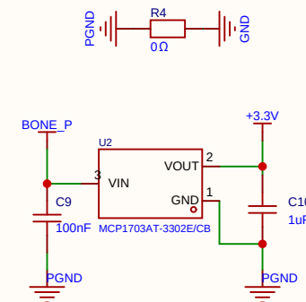
3.3V参考电压
