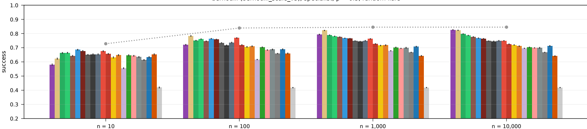
bernoulli (bernoulli_scale_v5), specialist, \beta = 0.5 , random liars
