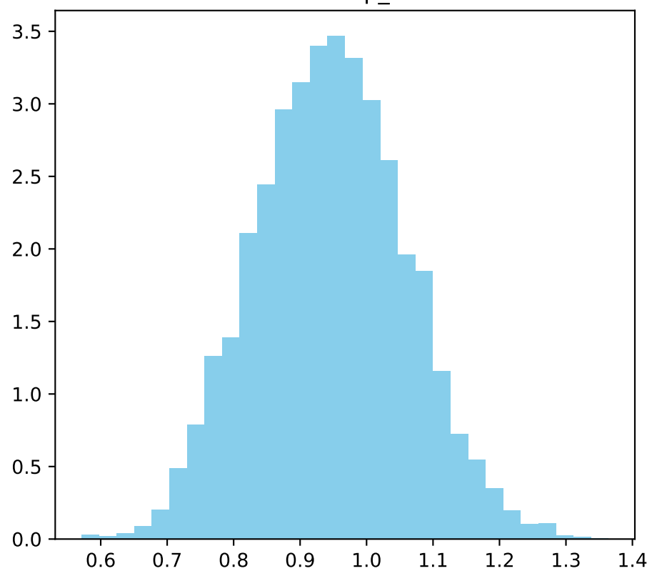
Posterior of \beta_{\text{Netflix}}
