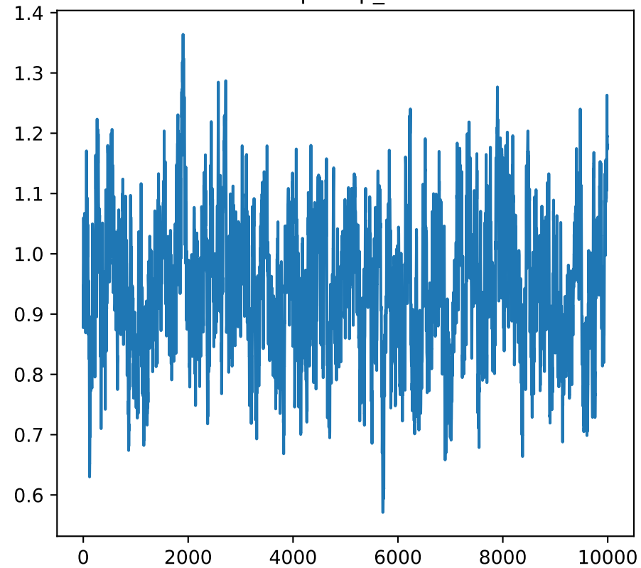
Trace plot: \beta_{\text{Netflix}}
