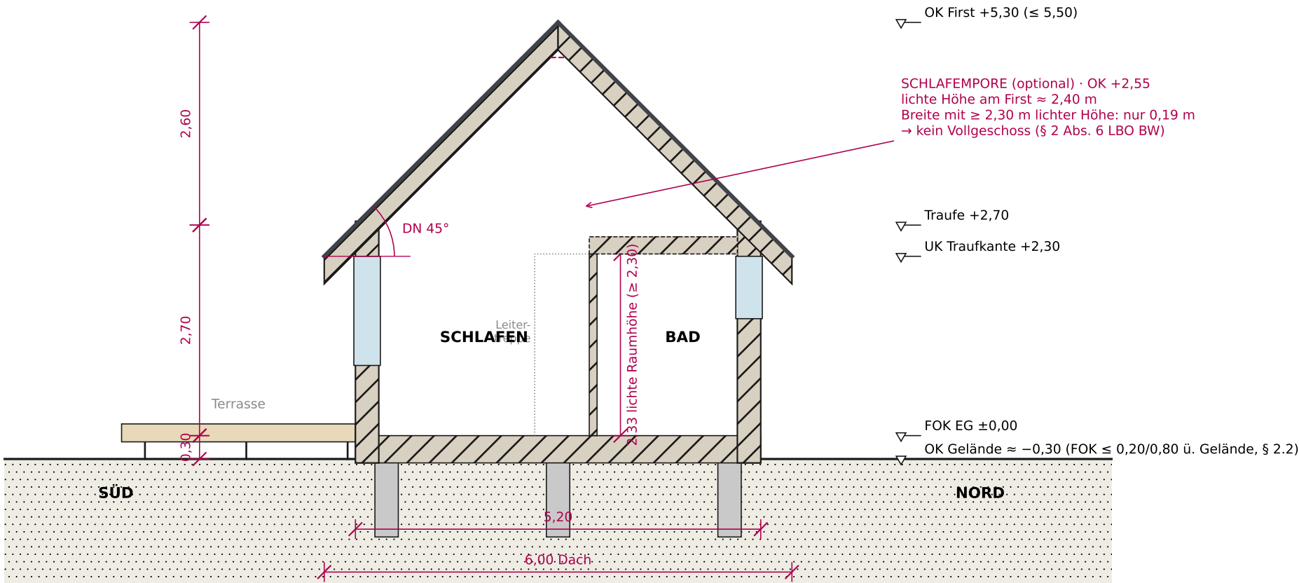
Punkt-/Schraubfundamente, frostfrei; Bodenplatte entfällt (Holzbalkendecke, hinterlüftet)
