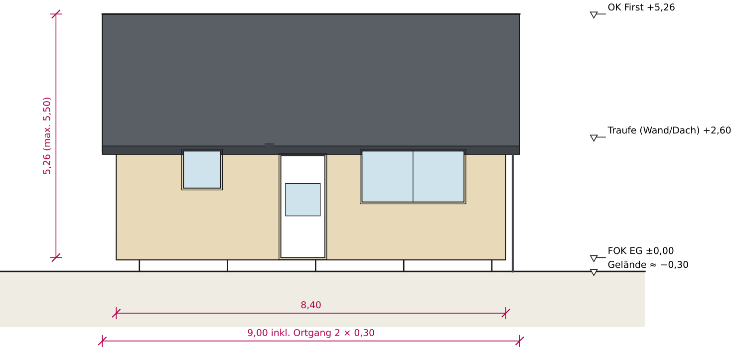
Ansicht Nord (Eingang / Grenzweg)
