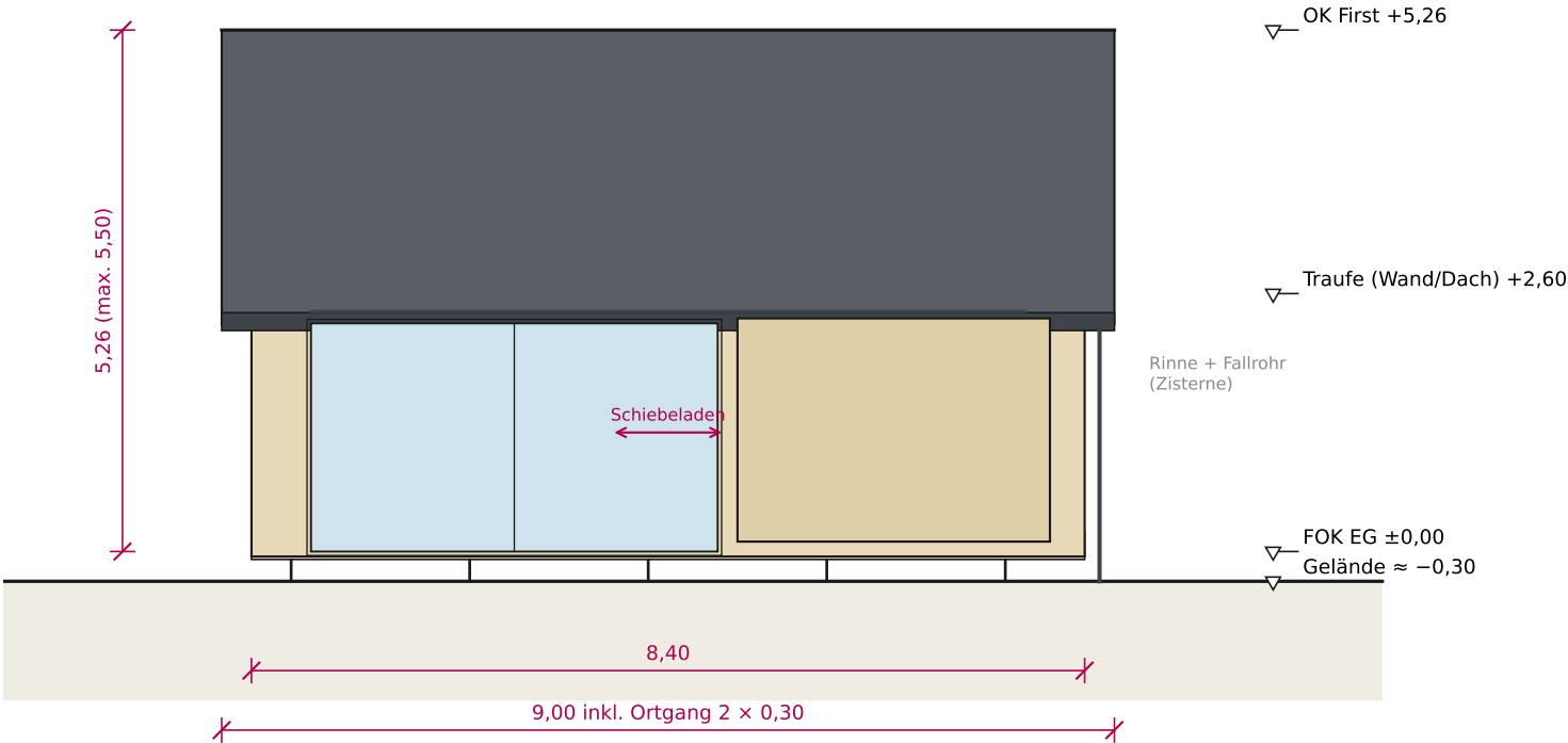
Ansicht Süd (Terrasse / Gartenseite)
