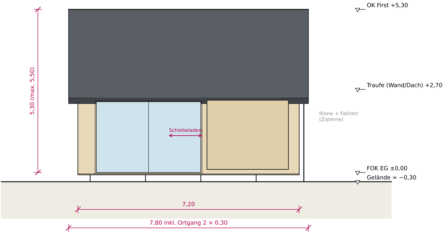
Ansicht Ost (Giebel, Waldseite)
