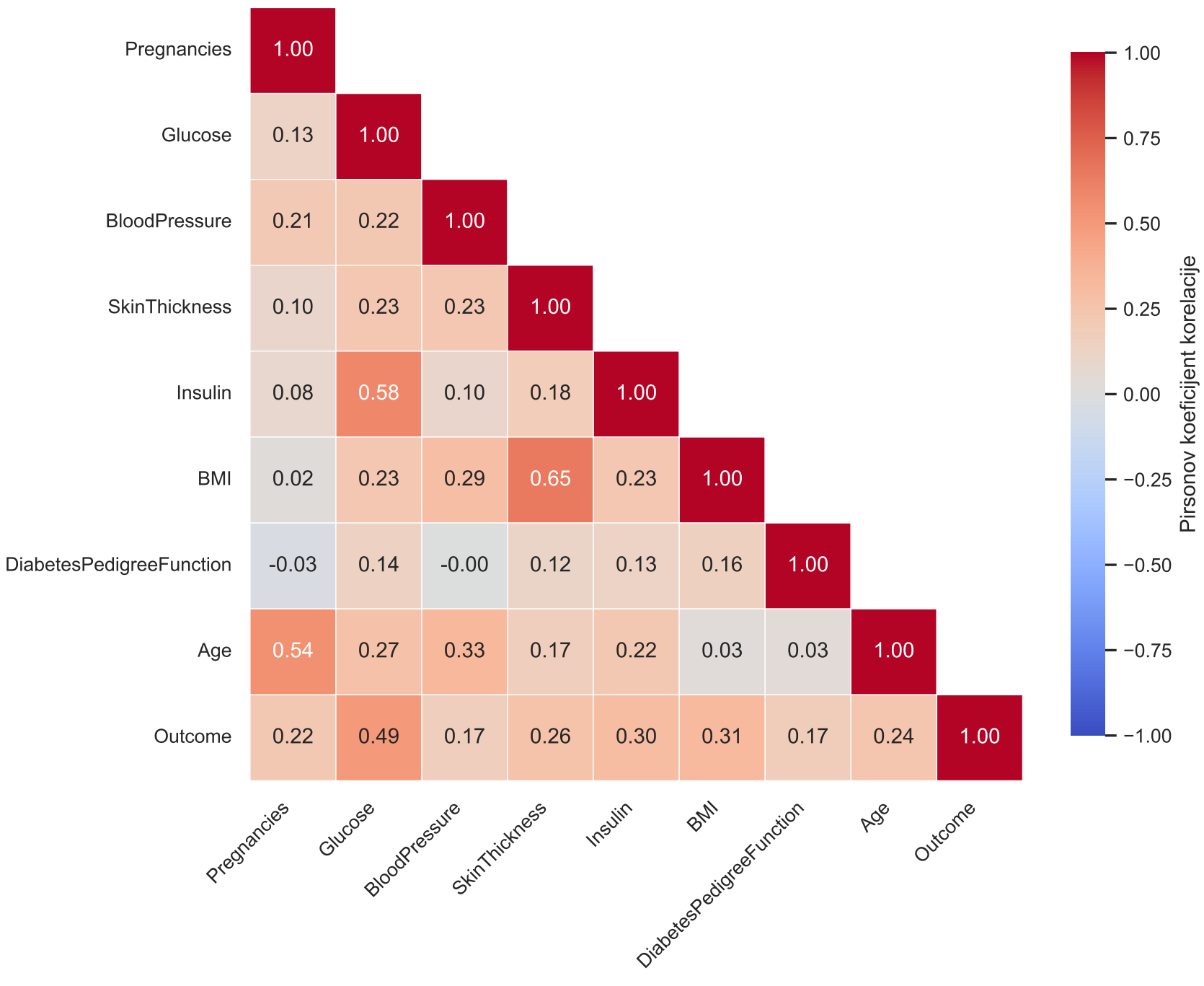
Korelaciona matrica atributa
