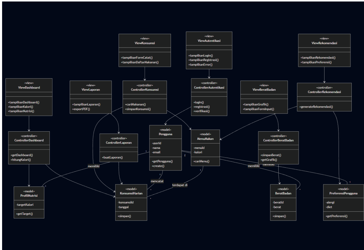
Gambar 3. 13 Diagram Kelas Keseluruhan
