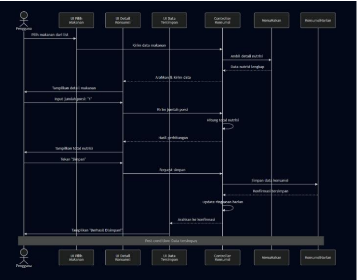
Gambar 3. 2 Seq Diagram#1 (Part 2): Input Detail Konsumsi & Simpan
