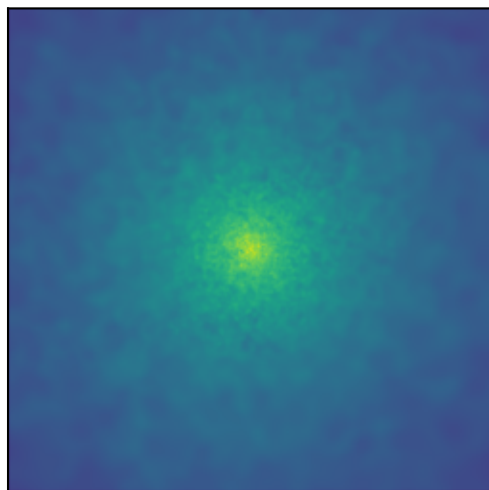
DM
