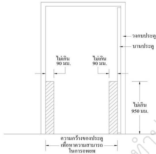
รูปที่ 5 ส่วนยื่นที่ยอมให้มีได้ในการวัดความกว้างของประตูเพื่อหาความสามารถในการอพยพ (ข้อ 1.5.2.2(2)(ข))
