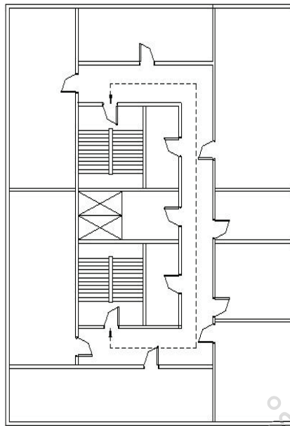
รูปที่ 3 การวัดระยะห่างของทางออกหนีไฟตามแนวช่องทางเดิน (ข้อ 1.4.4(4))
