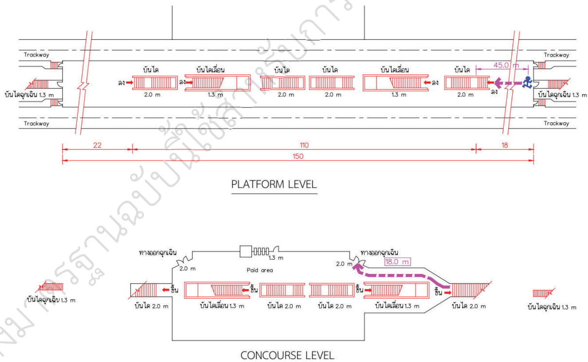
รูปที่ 23 สถานีชานชาลากลาง (center-platform station) (ข้อ 1.7.1)
