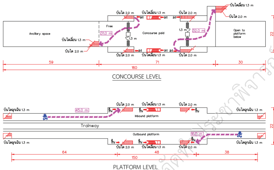
รูปที่ 24 สถานีขานขาลาข้าง (side - platform station) (ข้อ 1.8.1)
