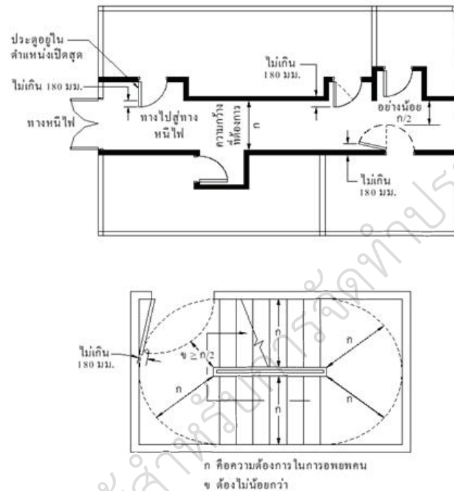
รูปที่ 7 ส่วนยื่นที่ยอมให้รับได้สำหรับช่องทางเดินและบันได (ข้อ 1.5.2.4(3))
