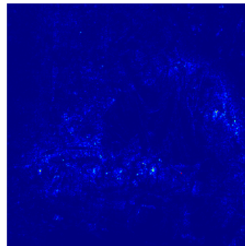
IG: Blur
