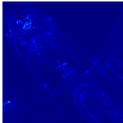
IG: Blur
