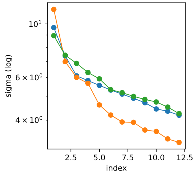
pool5 (C=512)
