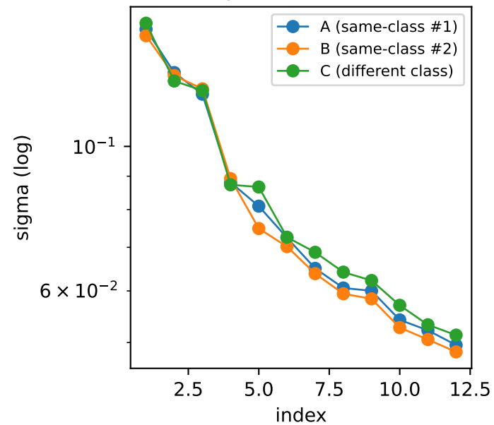
pool1 (C=64)
