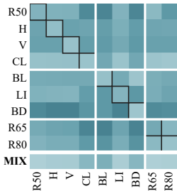
Poisson · U-FNO
