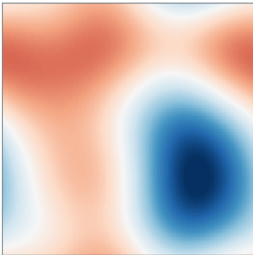
Poisson
