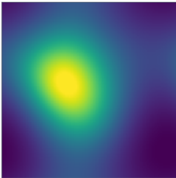
Darcy
