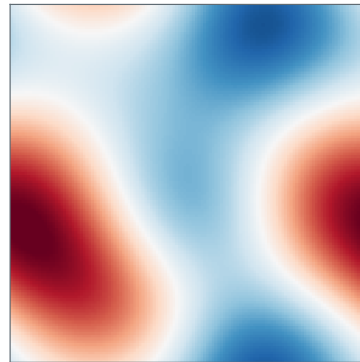
Reaction--diffusion
