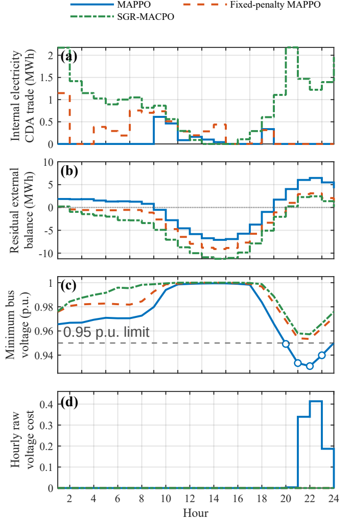
图 5: 代表性场景下从电力 CDA 到配电网的作用链: (a) 内部 CDA 成交量; (b) 清算后的外部剩余平衡量 (正值表示购电); (c) 馈线最低母线电压; (d) 原始电压成本。空心圆标记 MAPPO 的低电压时段。
