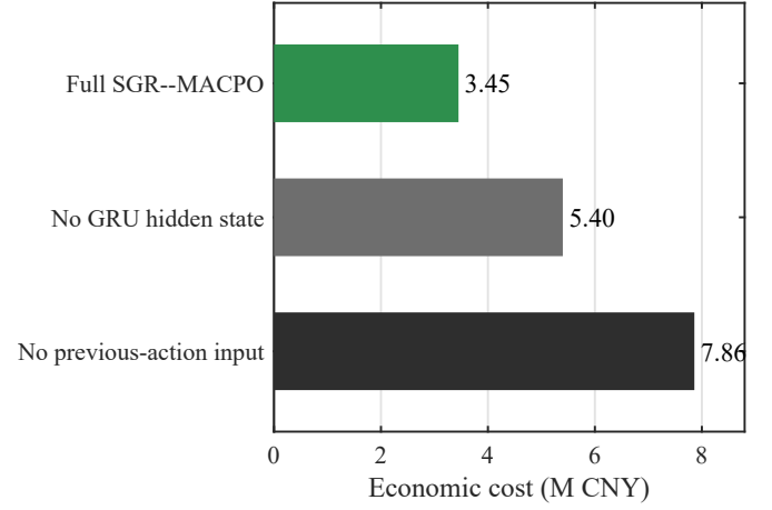
图 7: 代表性测试场景下基于同一检查点的循环信息消融实验。每次只移除图示时序输入, 其余策略参数和物理设置保持不变。
