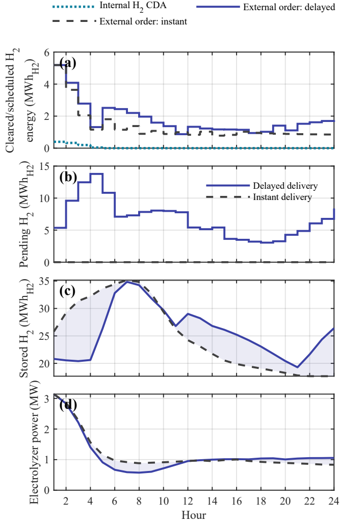
图 6: 代表性场景下延迟交付与即时交付两种情形的“氢气市场-物流交付”作用链: (a) 内部氢气 CDA 成交量及常规外购订单; (b) 在途待交付氢能; (c) 储存氢能; (d) 电解槽功率。实验仅改变实体交付时序, 策略检查点和观测维度保持不变。
