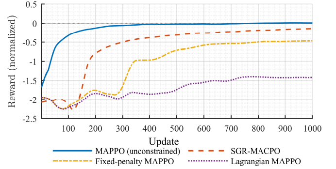
图 3: 各对比算法的缩放训练收益轨迹。为使单栏图中的安全-经济权衡更清晰, 收益曲线与电压成本曲线分别绘制。
