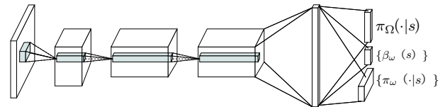
图6: 深度神经网络架构。将最后4张图像的拼接结果输入卷积层, 生成一个密集表示, 该表示在选项内策略、终止函数和选项上的策略之间共享。
