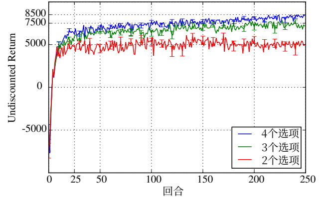
图5: 弹球领域中的学习曲线。
