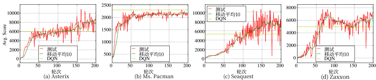
图8：街机学习环境中的学习曲线。所有四个游戏均使用相同的参数集：8个选项，0.01终止正则化，0.01熵正则化，以及选项内策略梯度的基线。
