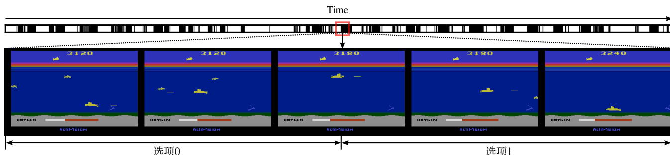
图9：在Seaquest中使用2个选项进行选项-评论家学习时发现的上下特化。顶部条带显示了游戏中的一条轨迹，其中“白色”表示选项1处于活动状态的片段，“黑色”表示选项2处于活动状态的片段。
