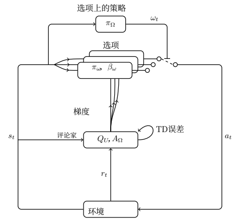
图1：选项-评论家架构示意图。选项执行模型通过一个开关 1 作用于触点 1 来描绘。仅当当前选项终止时，才会根据 \pi_{\Omega} 选择新选项。
