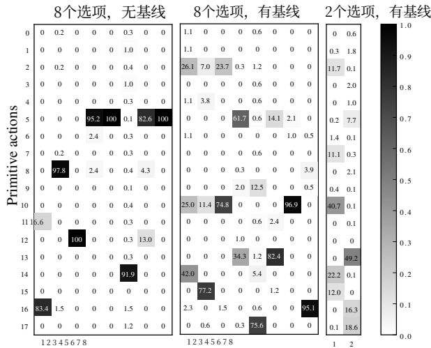
图7: Seaquest: 在梯度估计器中使用基线改善了选项内策略的动作分布，使其更少确定性。每列代表在Seaquest中学习到的一个选项。纵轴涵盖ALE的18个原始动作。经验动作频率通过强度编码。
