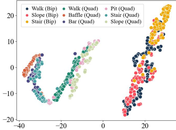
图8：门控网络在不同地形和步态下输出的t-SNE结果。
