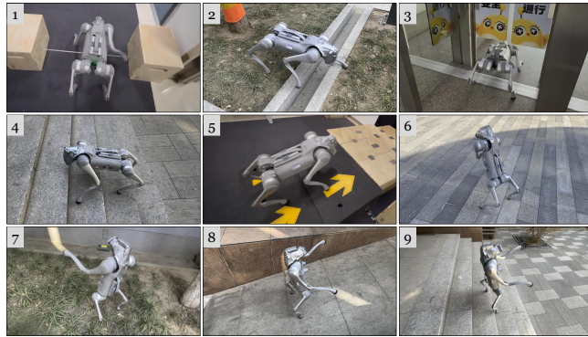
图5：多地形和多步态下的真实世界实验：1. 杆（四足），2. 坑（四足），3. 挡板（四足），4. 楼梯（四足），5. 斜坡（四足），6. 站立（双足），7. 行走（双足），8. 斜坡（双足），9. 楼梯（双足）。
