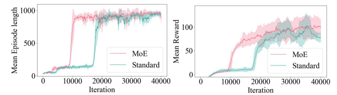
图6：我们的多任务策略在预训练阶段的训练曲线。
