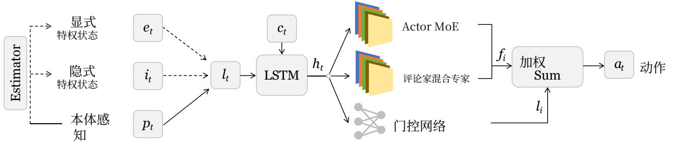
图3: 我们的MoELoco 流程概览。通过MoE架构的设计, 我们的策略在多种具有挑战性的地形上实现了稳健的多任务运动能力, 并支持多种步态。
