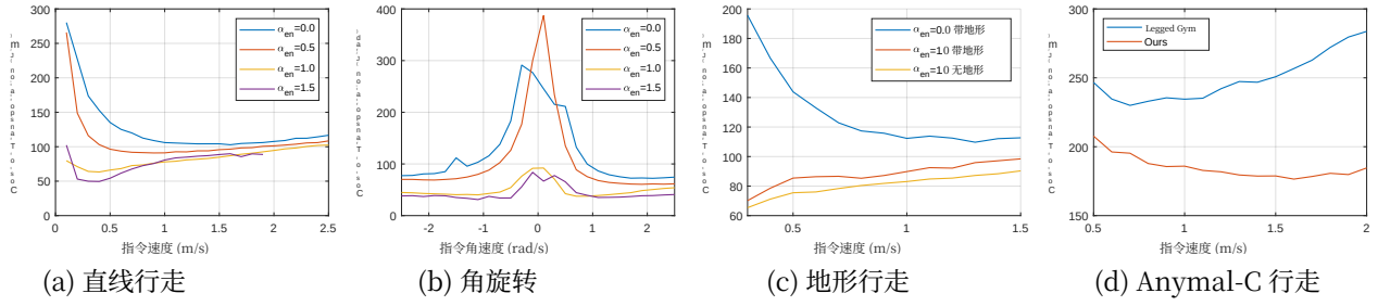
图 3: 宇树 Go1 仿真中能量消耗的消融研究。对于直线行走, 参考线速度从 0.1 到 2.5 m/s 选取, 间隔为 0.1。运输成本以 J/m 为单位测量。对于角旋转, 参考角速度从 -2.5 到 2.5 rad/s 选取, 间隔为 0.2。在 (a) 和 (b) 中, 当 \alpha_{en} 达到 1.0 时, 运输成本显著降低。当参考速度高于 1.9 m/s 时, \alpha_{en} = 1.5 的运输成本未绘制, 因为在此范围内输出速度降至零。这表明当能量正则化权重 \alpha_{en} 过大时, 速度跟踪精度会受到影响。对于地形行走, 机器人被要求在粗糙斜坡地形上直线行走, 参考线速度从 0.3 到 1.5 m/s 选取, 间隔为 0.1, 因为在此类地形上行走过慢或过快都很困难。(c) 显示运输成本的降低同样出现在地形上。(d) 展示了能量正则化方法对 ANYmal-C 平台的影响, 参数为 \sigma_{en,x} , \sigma_{en,z} 和 \alpha_{eno}
