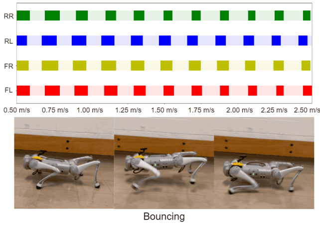
图4: 当 \alpha_{en}=0.0 时不同指令速度下的步态。该策略在所有指令速度下均表现为弹跳步态, 这不是一种节能的步态选择。我们还展示了弹跳步态的截图, 即四条腿几乎同时离地触地。
