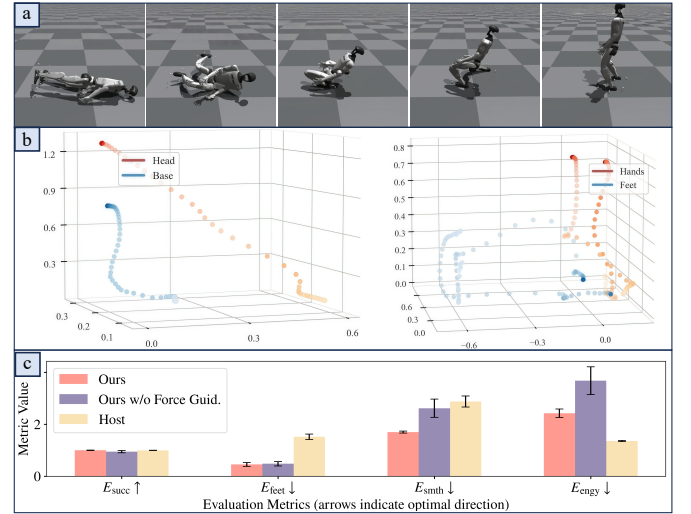
图5. 所提出的力引导方法已扩展至23自由度的宇树人形机器人。我们的方法学习了一种从任意姿态站立的策略(a)。恢复运动通过关键点的3D轨迹展示(b)，对比评估(c)证实了该策略的平滑性及其相对于其他方法的优越性。
