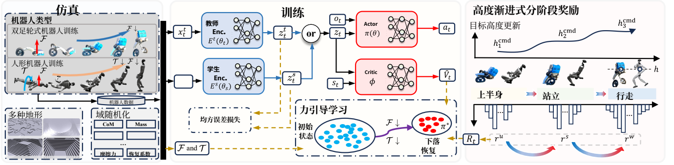
图2. 力引导跌倒恢复训练框架。该框架支持从“机器人类型”中选择双足轮式机器人或人形机器人。训练数据从所选机器人通过“机器人数据”流向教师编码器观测 x_t^t 和学生历史观测 o_{t:t-H}^s ，分别输入 E^t 和 E^s 以生成潜变量 z_t^t 和 z_t^s 。这些潜变量随后由“或”模块选择，其中 z_t^t 用于教师组智能体， z_t^s 用于学生组智能体，形成与 o_t 和 s_t 拼接的 z_t ，供共享的Actor-Critic网络（ \pi 和 \phi ）输出 a_t 和 \hat{V}_t 。在训练过程中，黄色箭头表示训练信号： z_t^t 和 z_t^s 通过均方误差损失监督 E^s ，而 \mathcal{F} 、 \mathcal{T} 、 R_t 和 \hat{V}_t 更新 E^t 、 \pi 和 \phi ，通过逐步减少 \mathcal{F} 和 \mathcal{T} ，以力引导学习方式使策略向 \pi^* 演化。随着机器人基座高度增加，当超过高度阈值的智能体达到智能体总数的三分之二时， R_t 从 r^u 过渡到 r^w ，使目标高度和奖励与实际高度进展同步。
