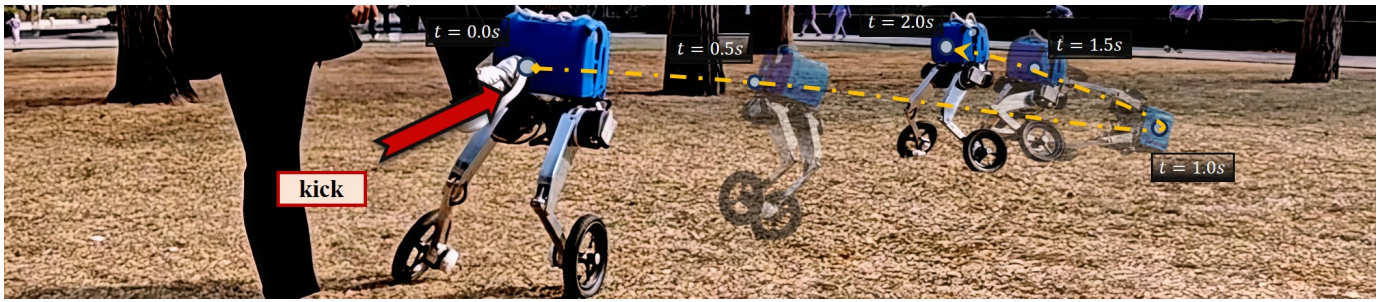
图8. 跌倒恢复及后续运动测试。外部踢击的方向用红色箭头标记，而实验过程中机器人基座的轨迹用黄色虚线箭头表示。结果表明，我们的方法能够自主从跌倒中恢复并继续执行运动指令。
