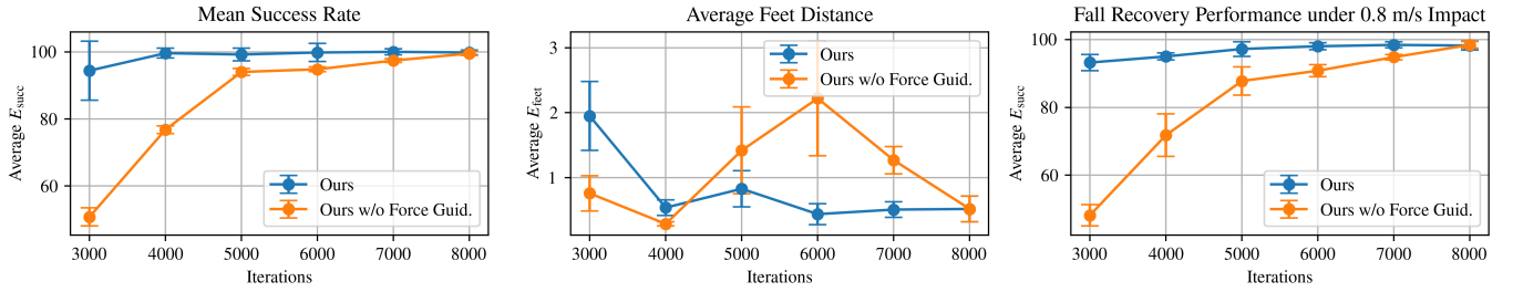
图4. 训练迭代中的成功率和足部移动距离。与无力基线相比，我们的力引导方法在3k次迭代时实现了高恢复成功率，并在4k次迭代时获得了更高的稳定性。这些结果证明了快速收敛和有效性所提出的力引导方法的有效性。
