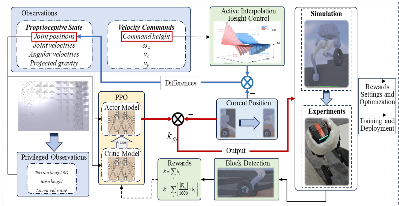
图2. 使用PPO的机器人系统高度控制框架。系统接收本体感受状态和特权观测以生成速度指令。由演员和评论家网络组成的PPO模型处理这些输入，为高度控制提供主动插值。该系统在仿真和真实场景中均得到验证，并通过奖励评估性能。输出：使用PPO算法优化后，演员模型输出的位置与当前位置之间的差值作为控制输出。差值：定义为插值后的大腿和膝关节角度与机器人当前构型角度之间的偏差。
