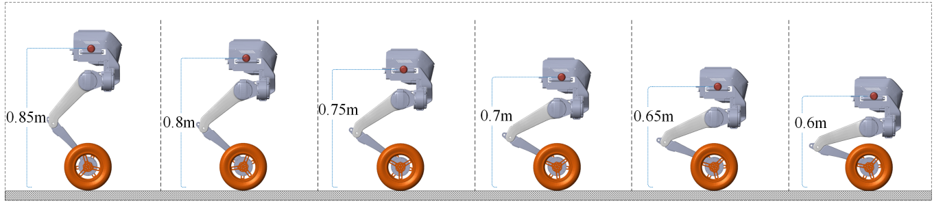
图4. 预设高度-关节角度映射关系。
