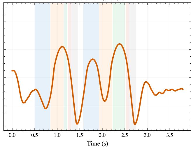
(d) VMC+SRL
