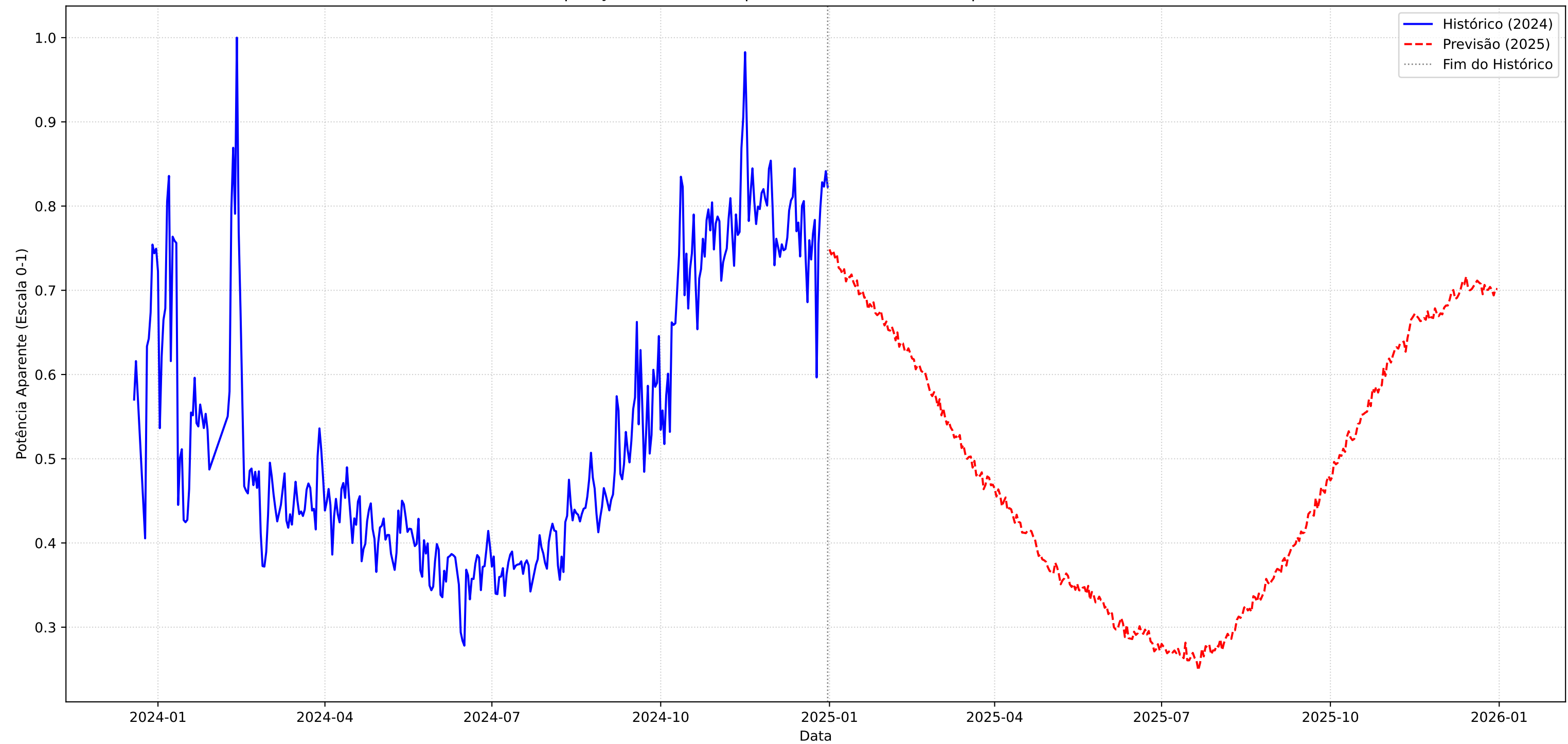
Extrapolação da Demanda para 2025 - LSTM Multi-Output (H=365) - T1
