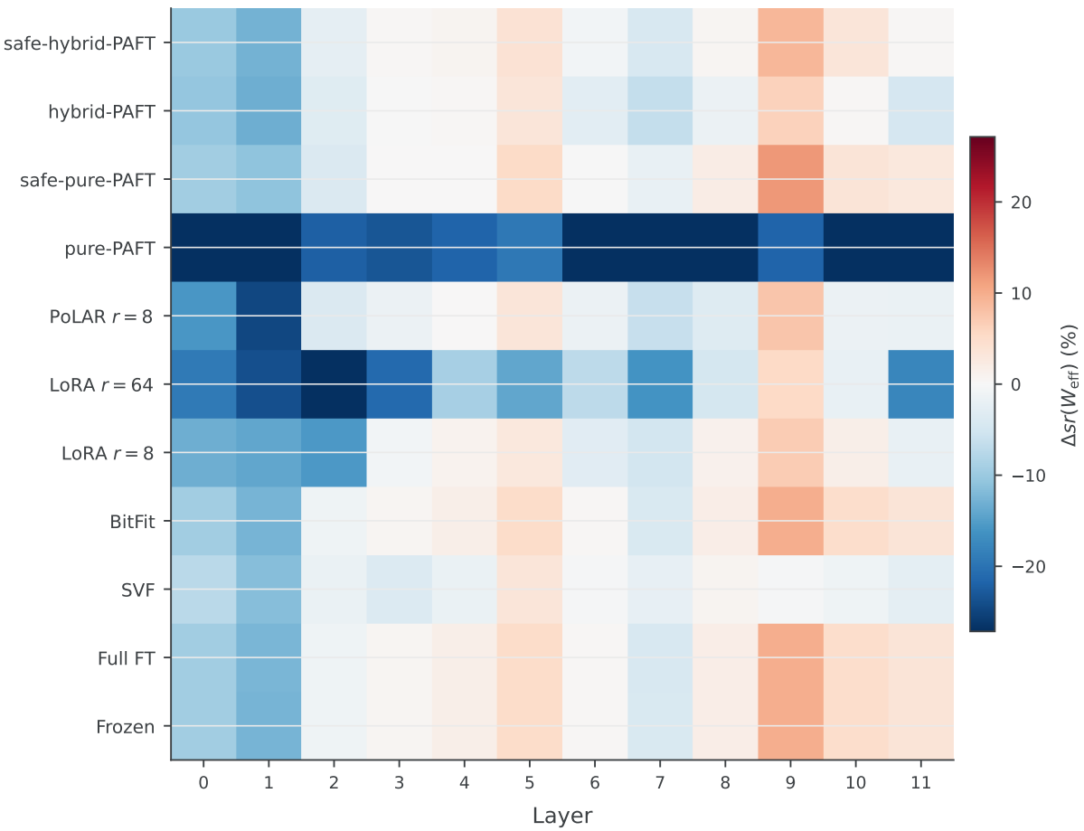
STS-B
