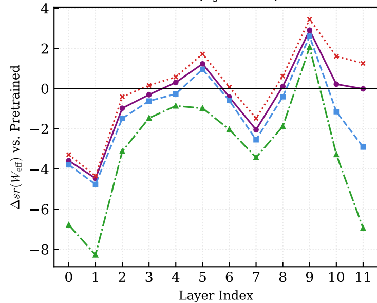
CoLA (Syntactic)
