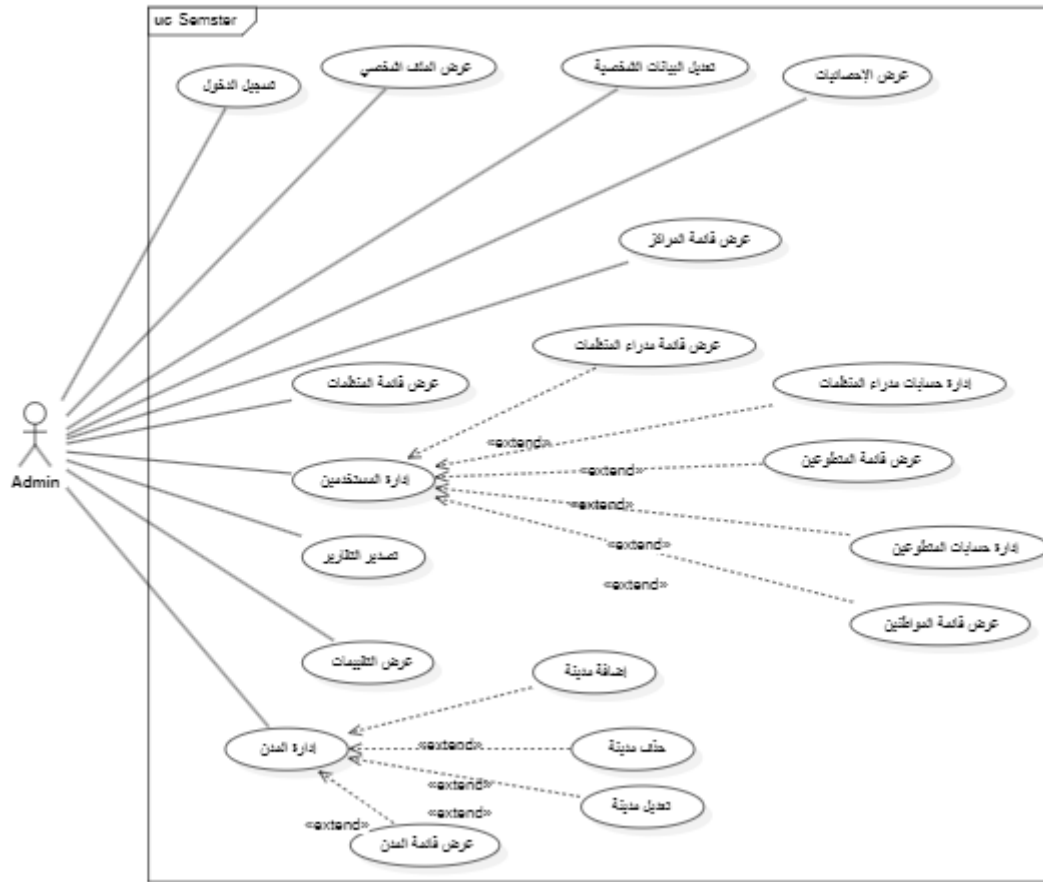
الشكل (2.2) مخطط حالات الاستخدام التي تم العمل عليها في المشروع الفصلي
